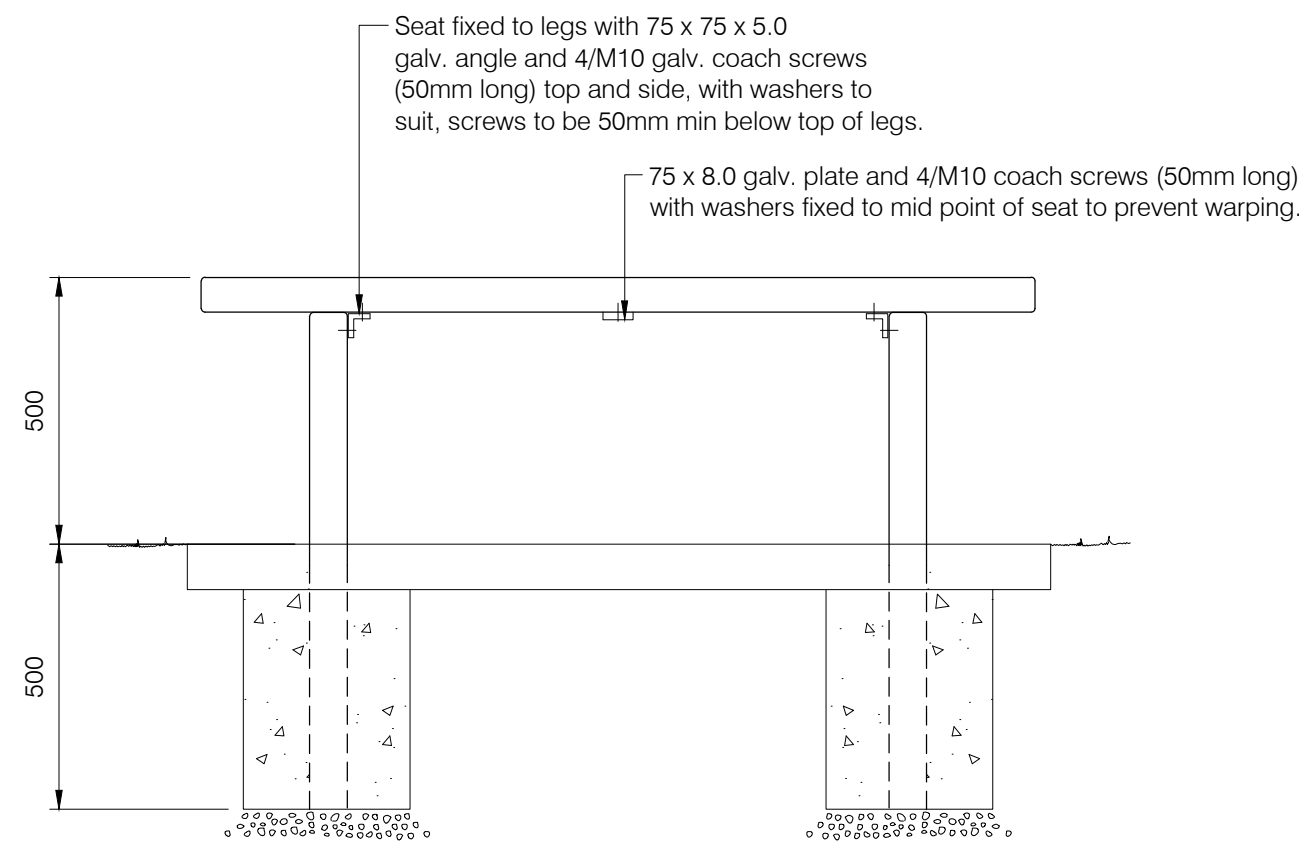
ELEVATION
